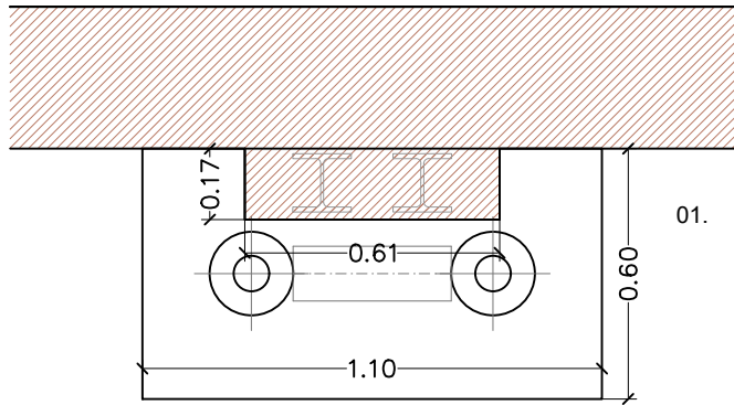
01. CONSTRUCCIÓ D'ENCEPAT ARMAT AMB DOS MICROPILOTS SOTA PILASTRA PER SUPORT DE FUTURS PERFILS I RECALÇ DE PARET EXISTENT
