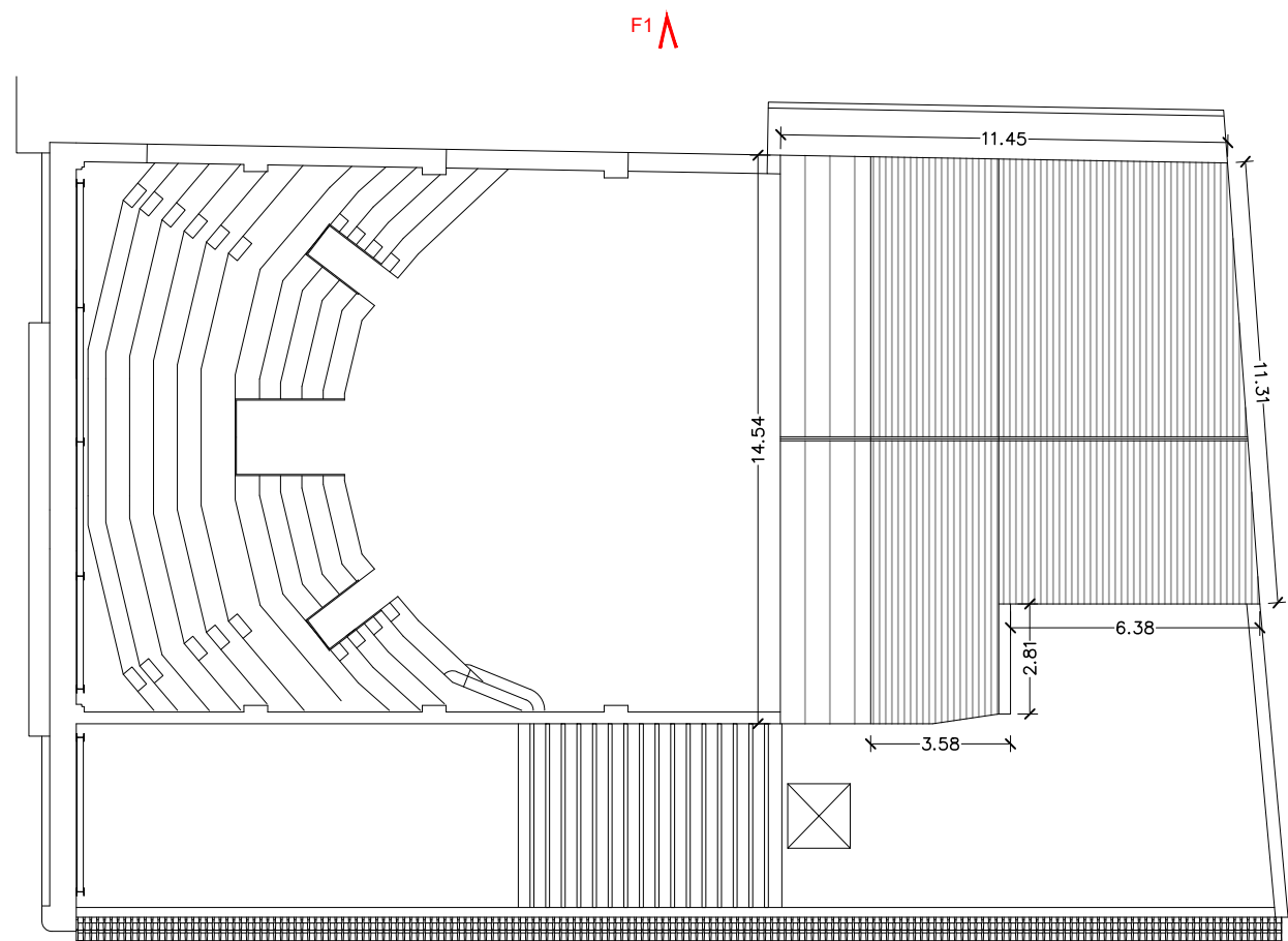
PLANTA COBERTA
