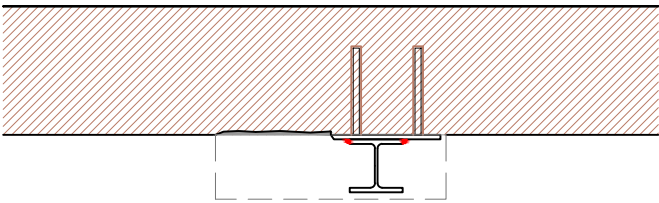
05. RETALLAR RESTA DE PILASTRA I REGULARITZACIÓ DE LA PARET AMB MORTER
