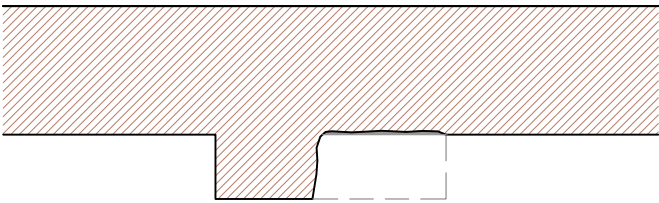
02. RETALLAR PILASTRA PREVI APUNTALAMENT DE PARET I REGULARITZACIÓ DE LA PARET AMB MORTER REALITZAR OPERACIÓ PER TRAMS DE 3m DE DALT CAP A BAIX (CONJUNTAMENT AMB EL PAS 03)
