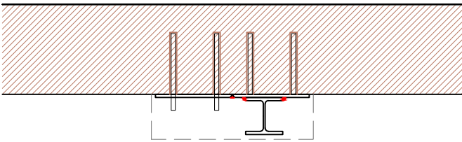
06. COL.LOCACIÓ DE XAPA METÀLICA ANCORADA A LA PARET AMB BARRS ENCASTADES AMB RESINES XAPA BISELLADA PER FUTURA SOLDADURA SOLDAT DE LES XAPES ANCORADES A PARET
