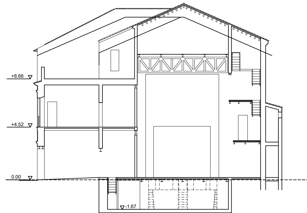
SECCIÓ TRANSVERSAL 1
