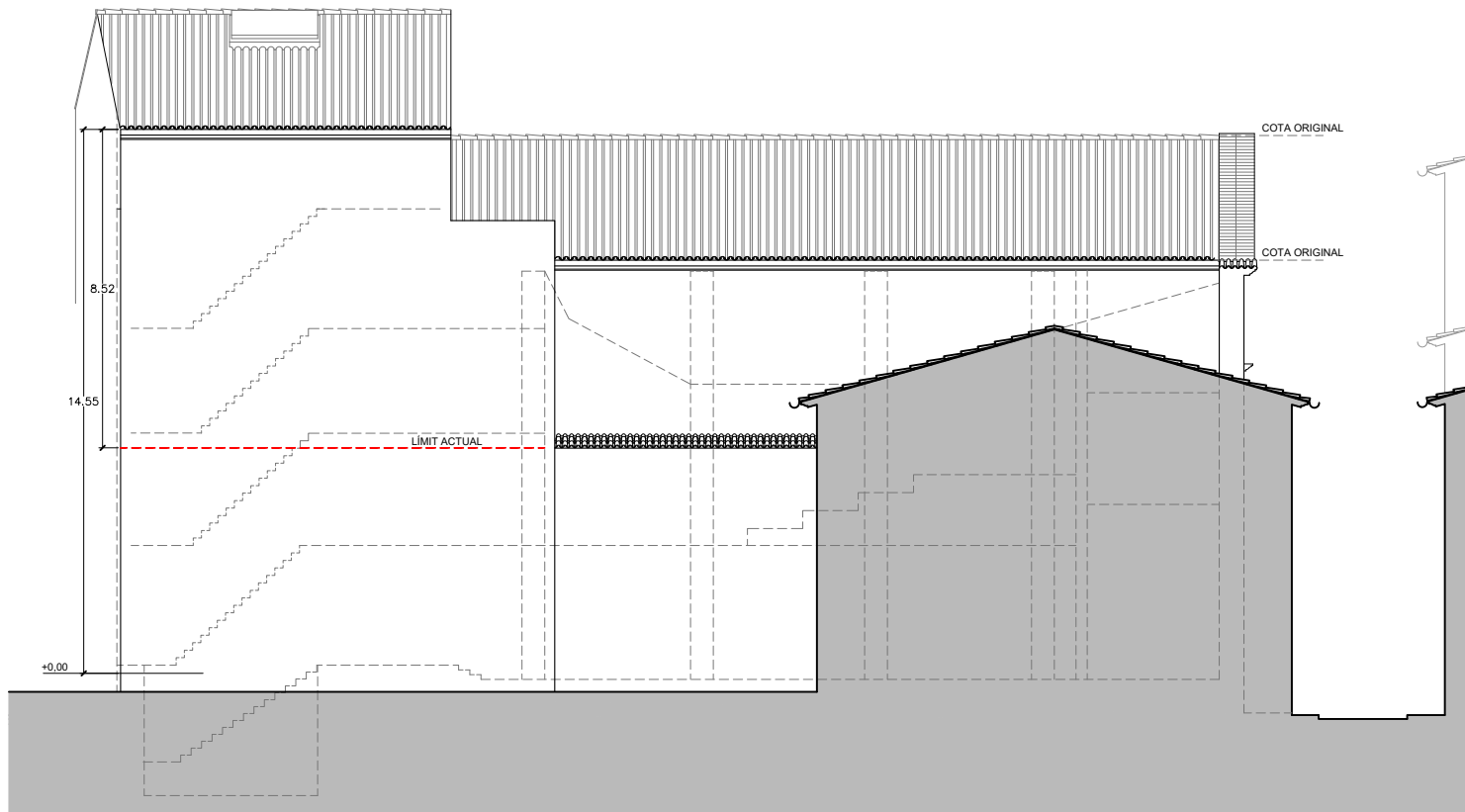
ALÇAT 3 MITGERA LATERAL
