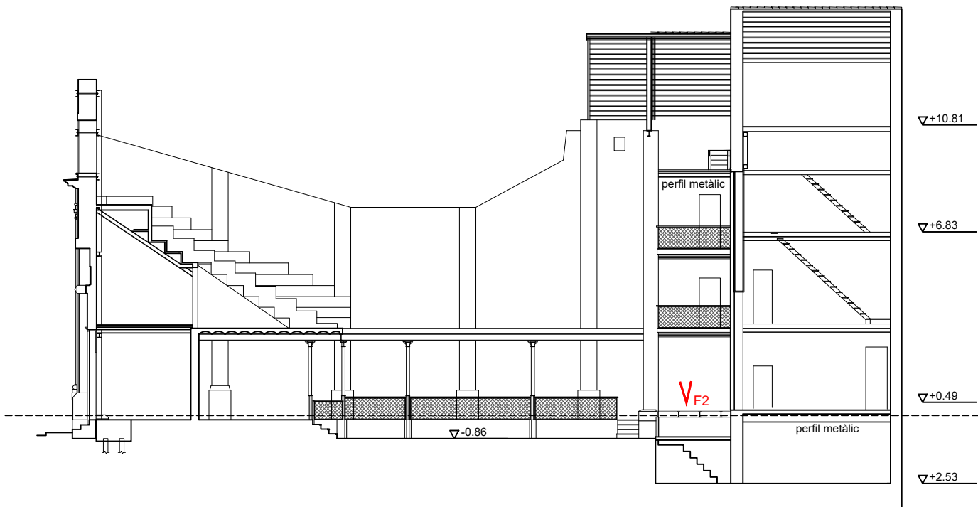
SECCIÓ LONGITUDINAL 2
