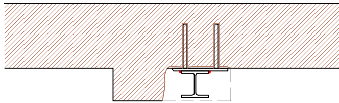
04. COL.LOCACIÓ DE HEB140 SOLDADA A LA PLACA
