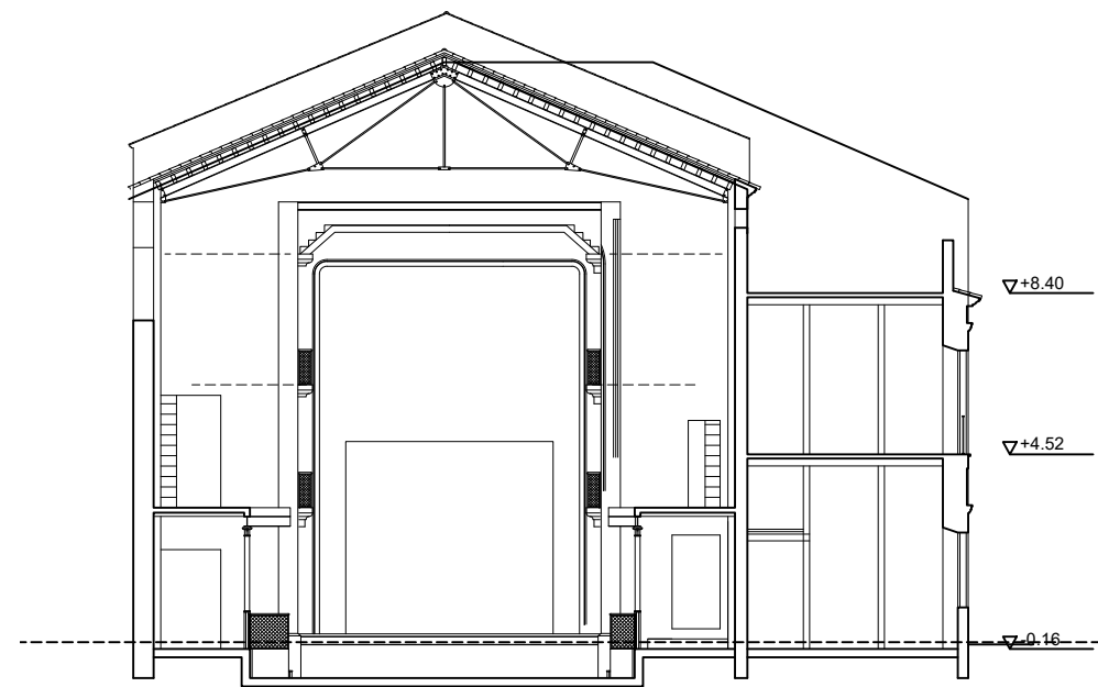
SECCIÓ TRANSVERSAL 1
