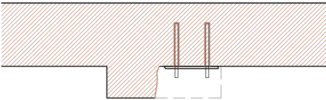
03. COL.LOCACIÓ DE XAPA METÀLICA ANCORADA A LA PARET AMB BARRS ENCASTADES AMB RESINES XAPA BISELLADA PER FUTURA SOLDADURA
