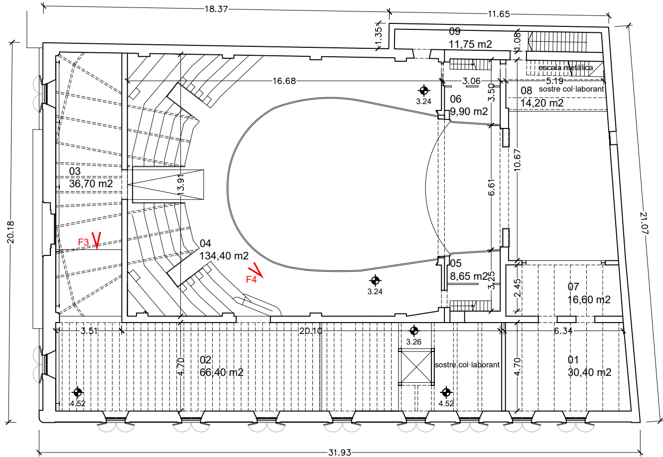
PLANTA PRIMERA
