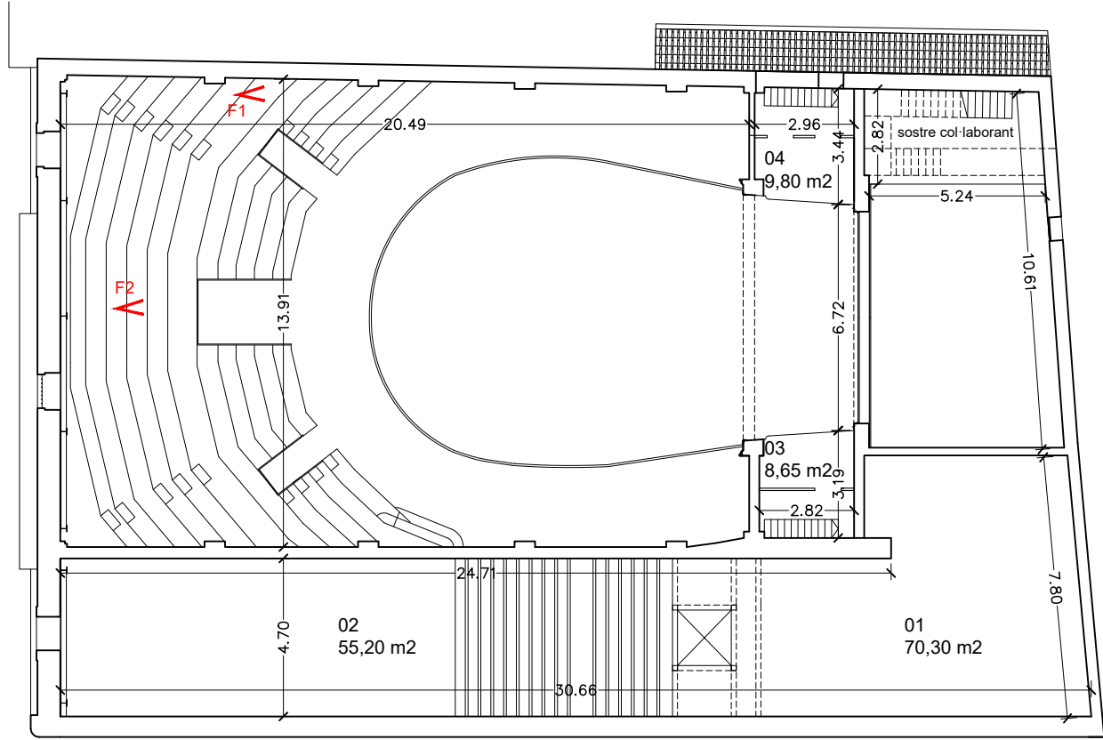
PLANTA SEGONA
