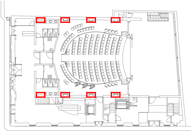
07. COL.LOCACIÓ DE SEGONA HEB140 SOLDADA A LA PLACA
