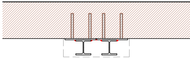
07. COL.LOCACIÓ DE SEGONA HEB140 SOLDADA A LA PLACA
