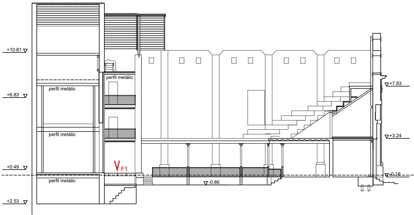
SECCIÓ LONGITUDINAL 1
