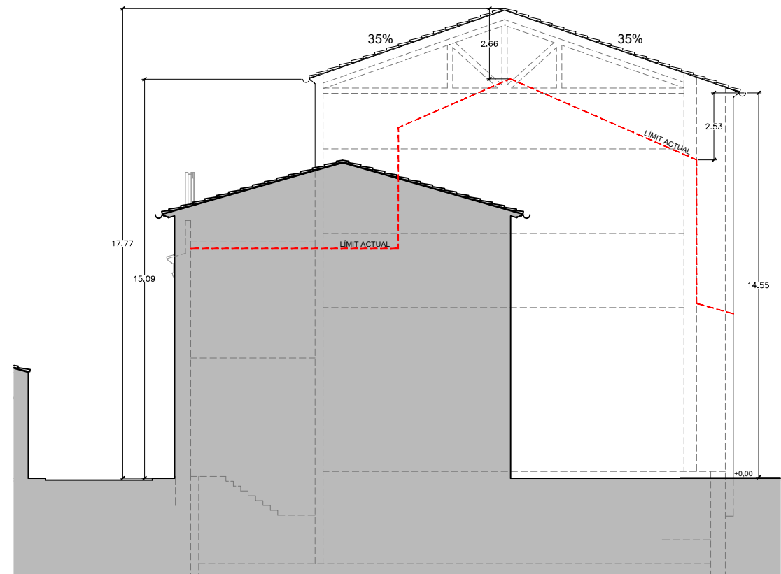
ALÇAT 4 MITGERA ESCENARI
