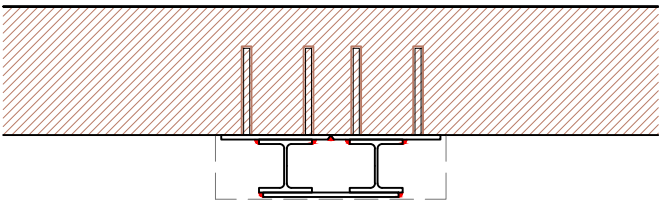
08. COL.LOCACIÓ DE XAPES METÀL·LIQUES SOLDADES A LES HEB140
